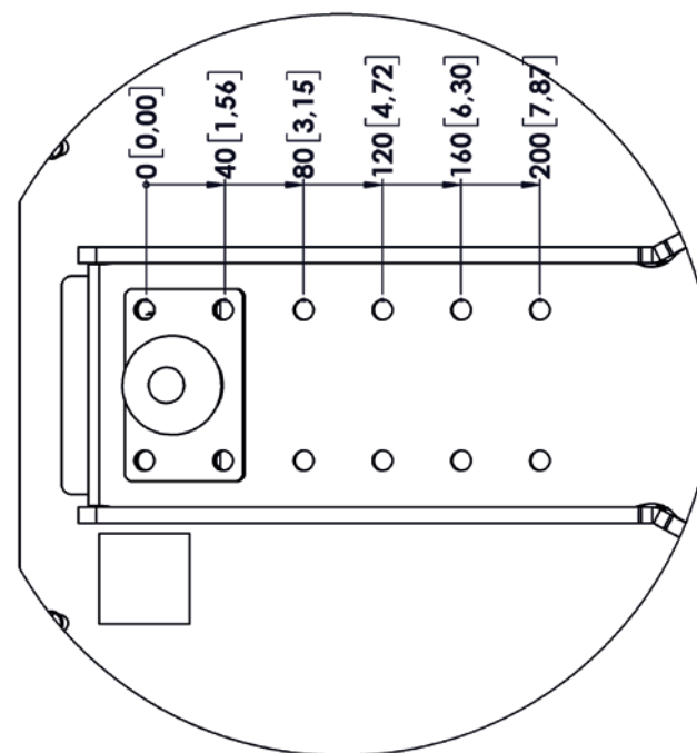
DETTAGLIO A SCALA 1:3
